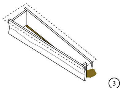
Schéma de restitution de l'effondrement du coffrage (au 1/50)
